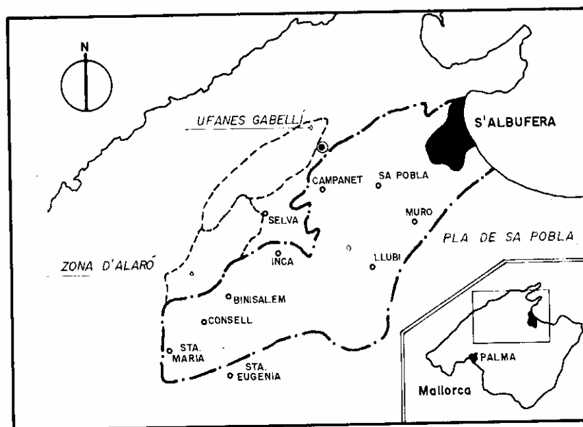
Croquis 3. Àrea de recarrega de l'aqüífer de Sa Pobla (Ullals de S'Albufera), i altres que aporten aigua subterrània indirectament al Parc.
